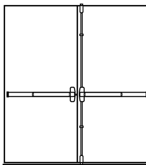
Puertas de Doble Hoja sin Paral Central Barra Horizontal + Barra Vertical + Cantonera especial
